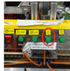
8. PINDUTIN ANG UP BOTTON PARA UMANGAT ANG LAGAYAN NG STRAP BELT
